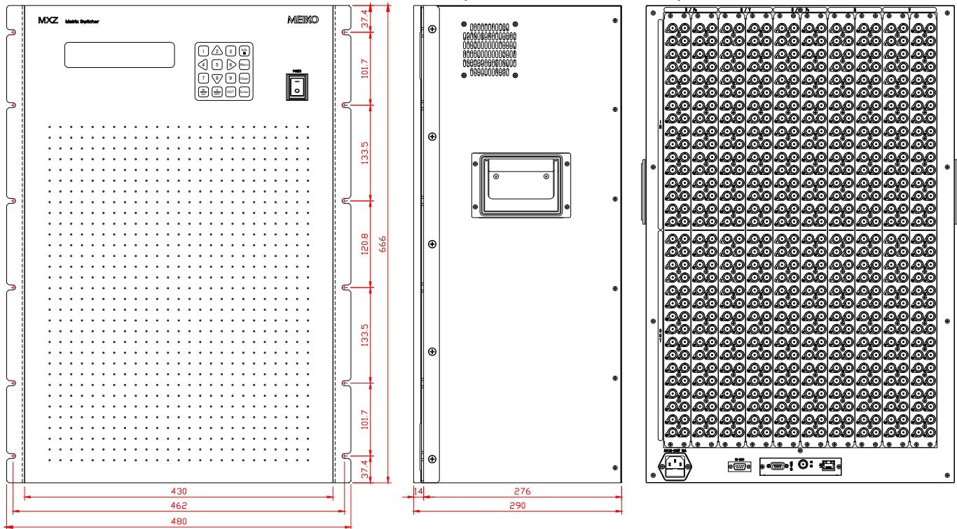
MXZ64-64R (ラックマウント金具実装図)
