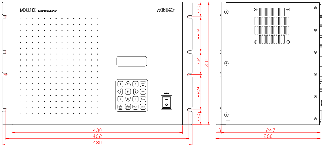
MXU 16-16DA (ラックマウント金具実装図)
