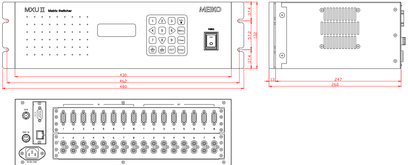
MXU 8-8DA (ラックマウント金具実装図)
